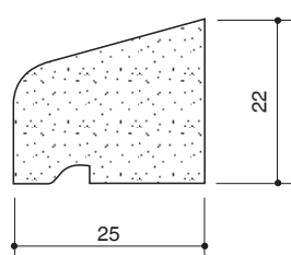
Art. Nr. 70.158.11 Wasserschenkel
