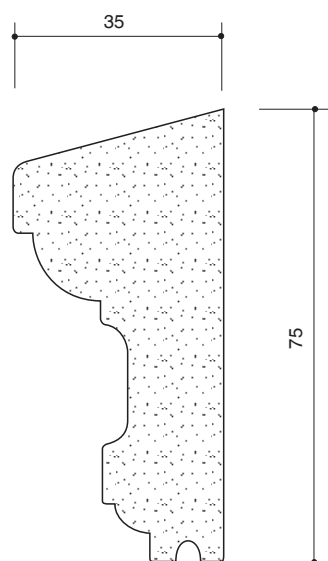
Art. Nr. 7015011 Zierleiste
