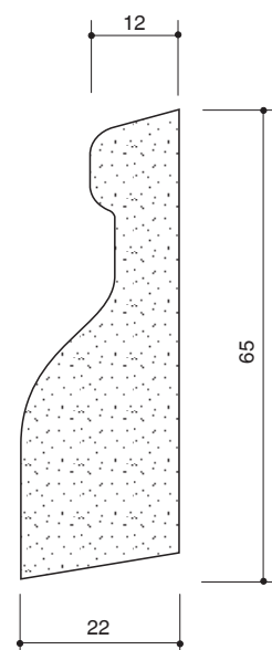
Art. Nr. 7016011 Zierleiste
